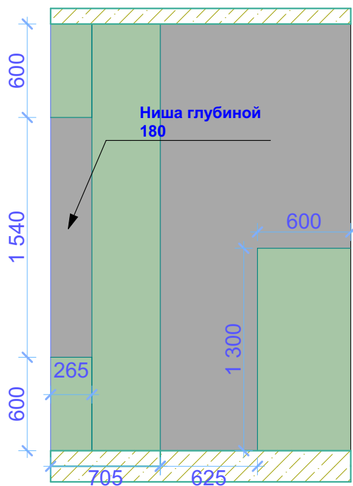
Разрез 2 Санузел
